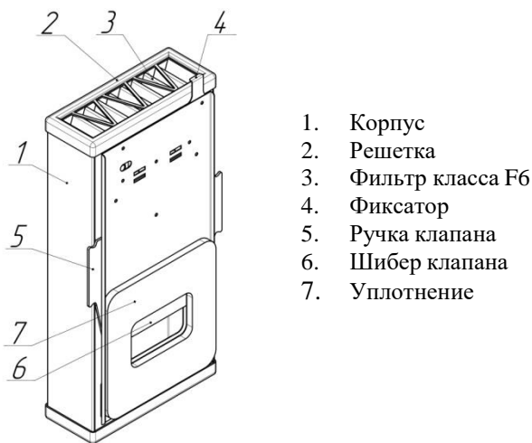
Рис. 3 Устройство шумоглушителя
